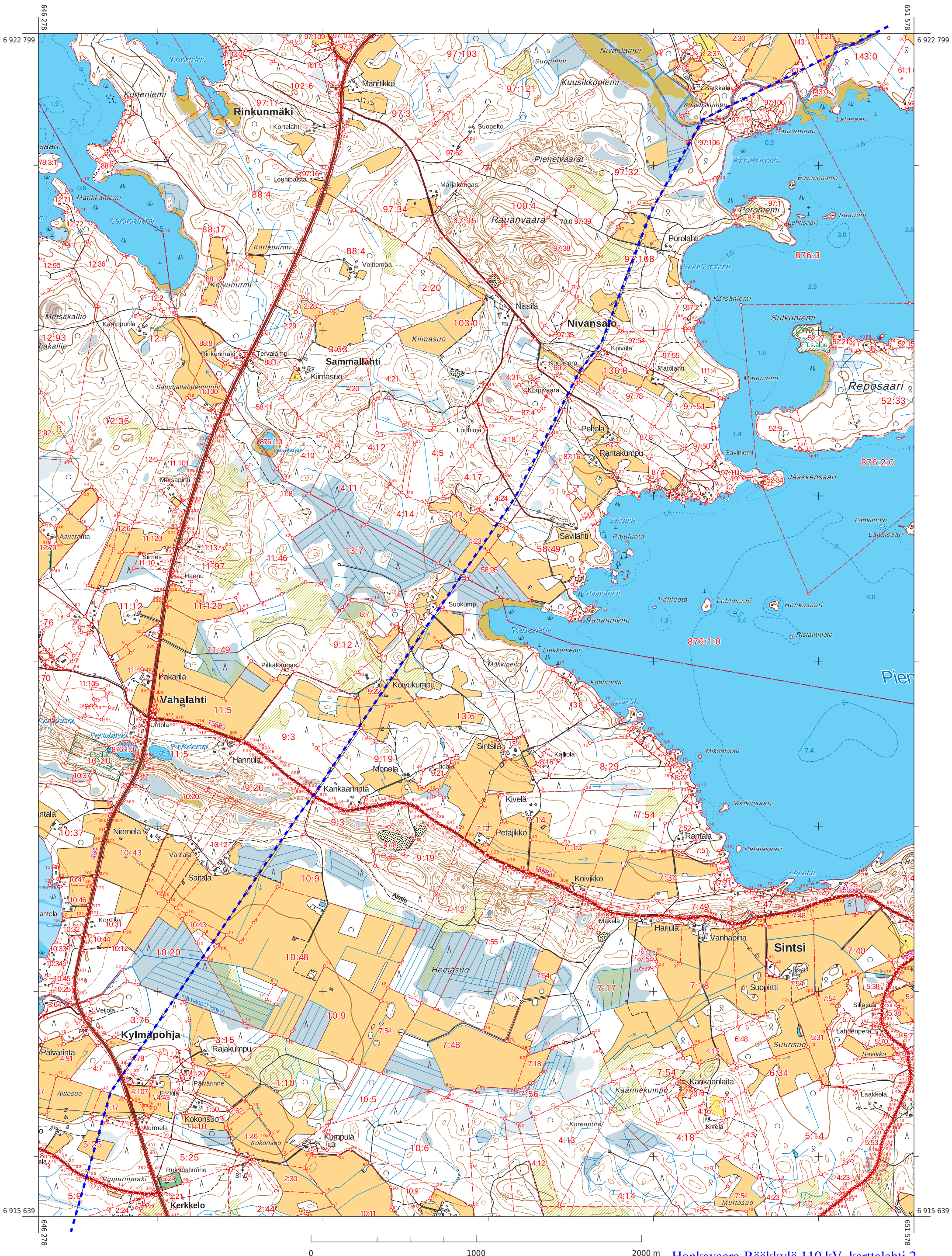
Honkavaara-Rääkkylä 110 kV, karttalehti 2
