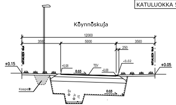
Pääliysrakenne / Katuluokka 5
