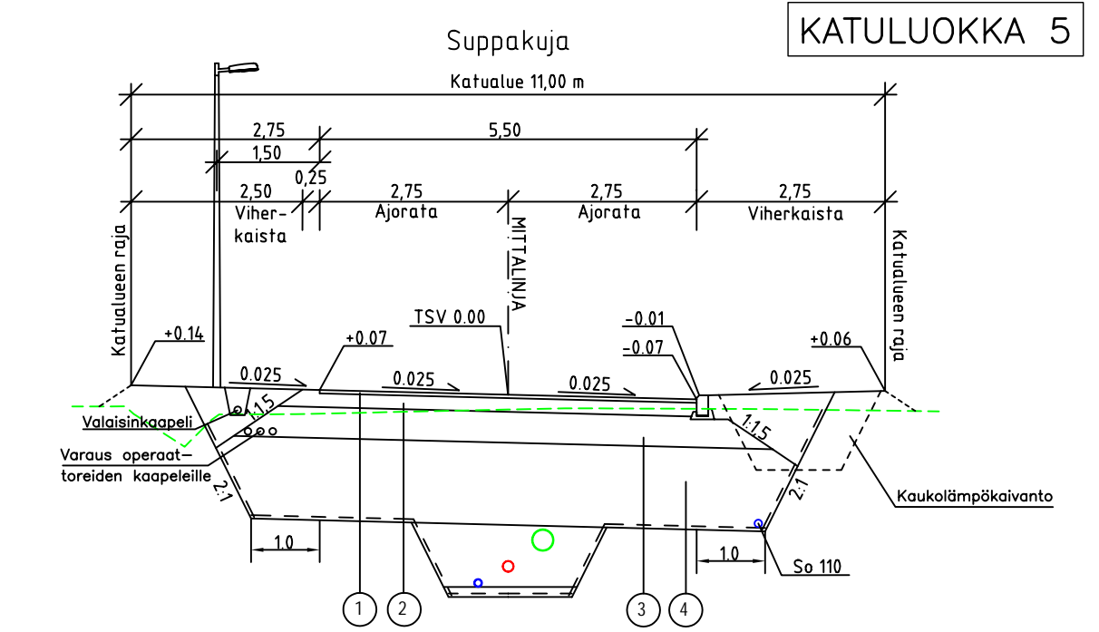
PÄÄLLYSRAKENNETAULUKKO AJORATA
