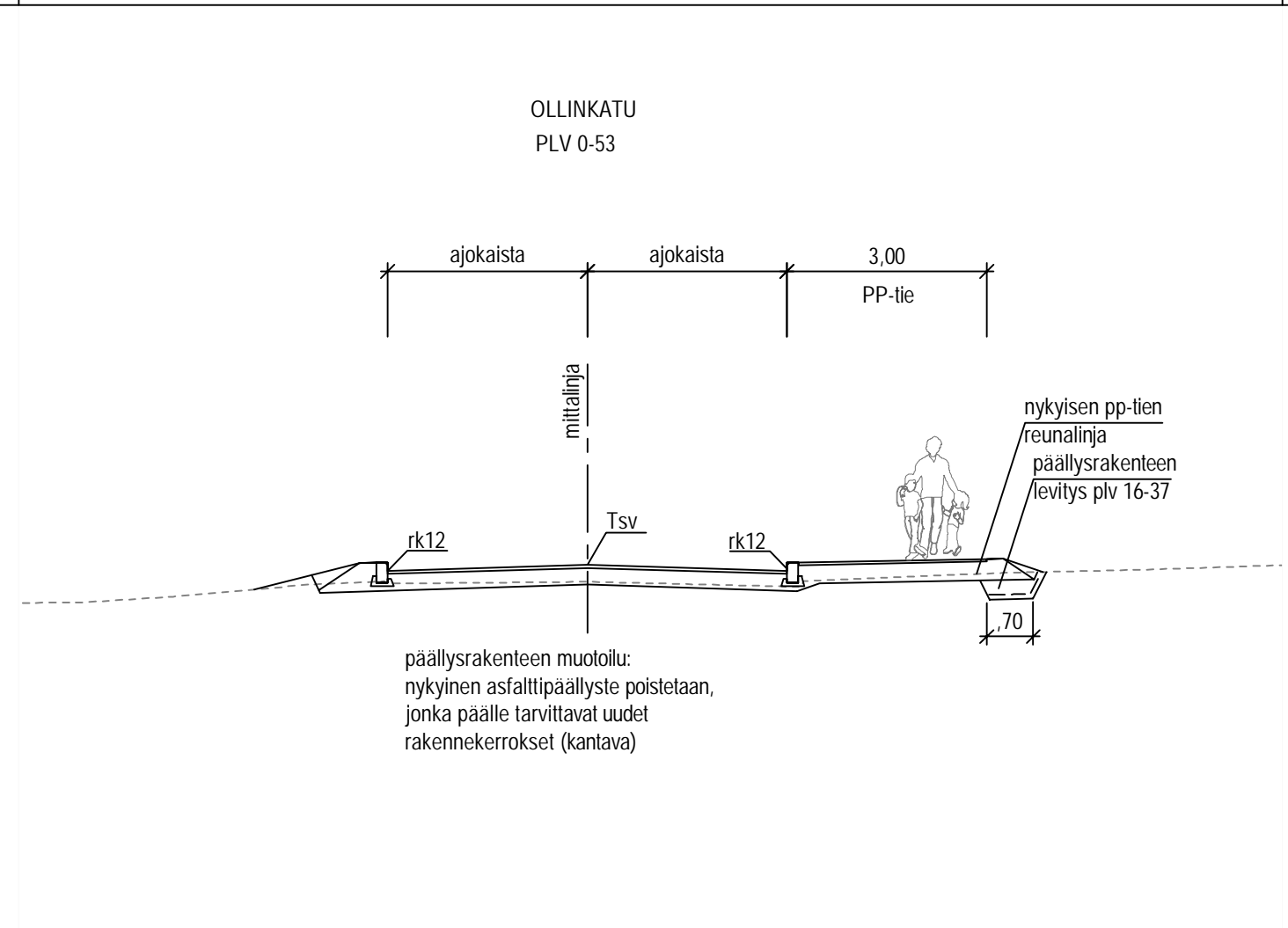
PÄÄLLYSRAKENNETAULUKKO, AJORATA
