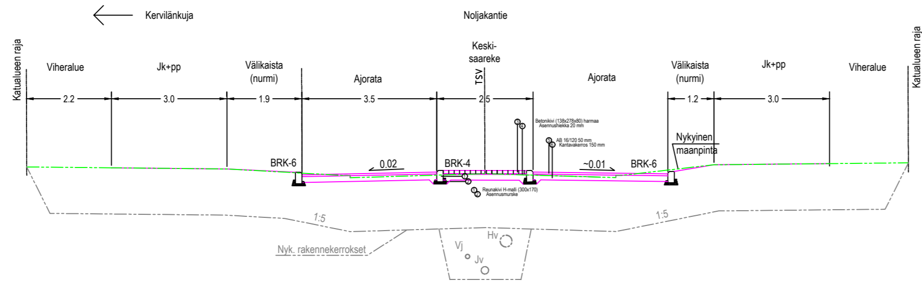
Jk+Pp, arvioitu nykyinen päällysrakenne Päällysrakennetaulukko / Katuluokka 6
