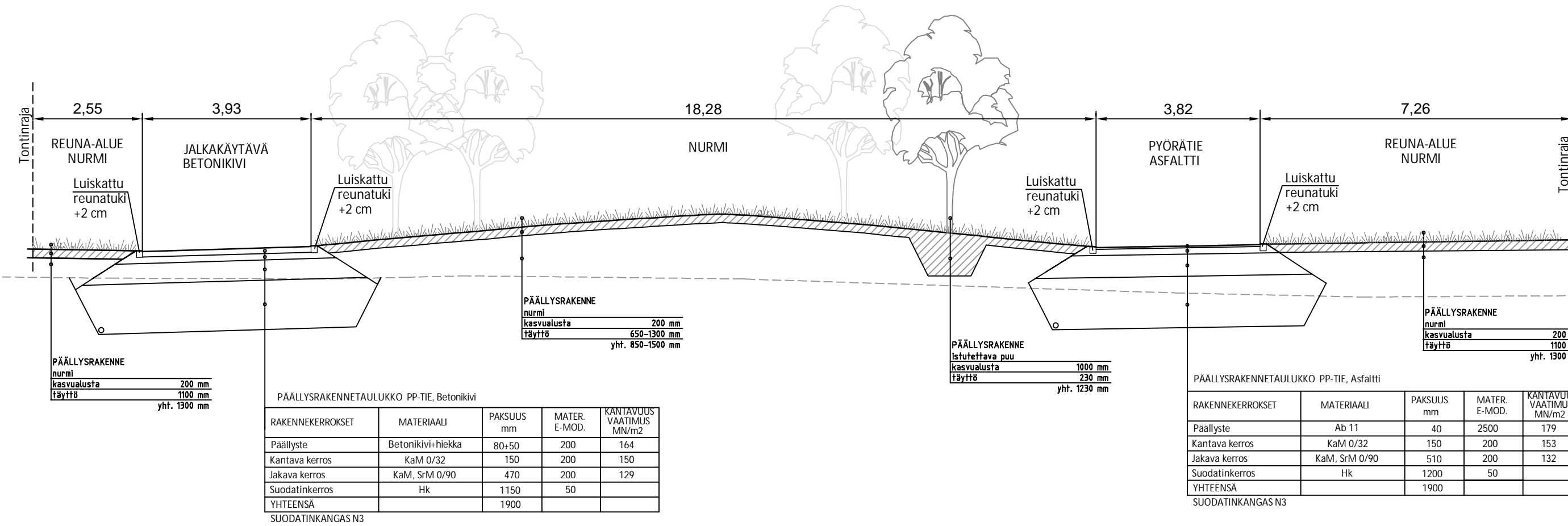
Leikkaus A-A, 1:100
