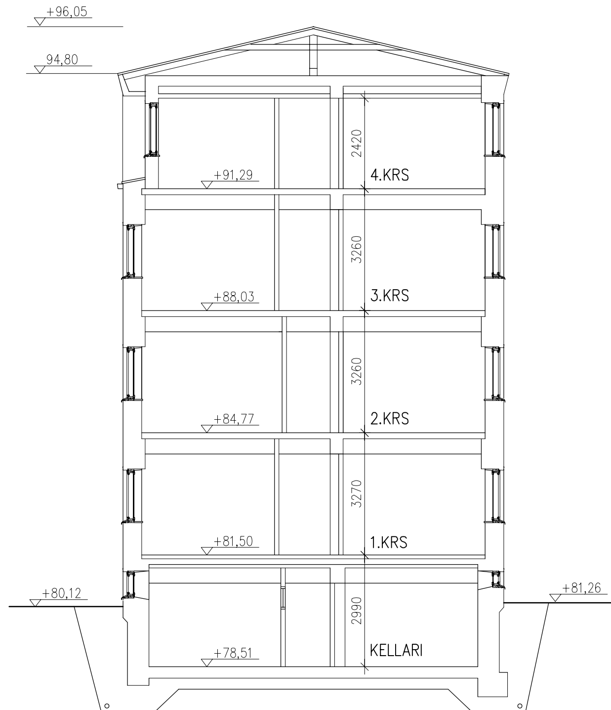
LEIKKAUS 3-3
