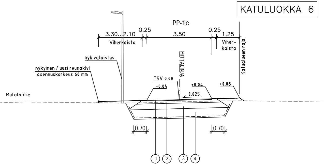
PÄÄLLYSRAKENNETAULUKKO PP-TIE
